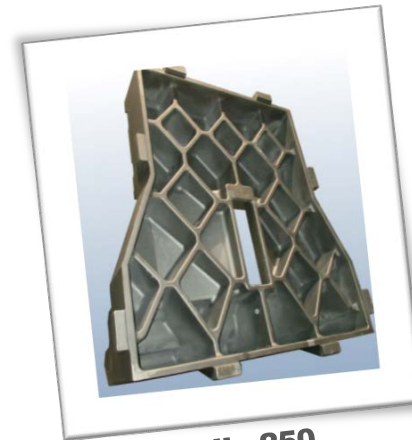
EN-GJL -250 1540 kg
